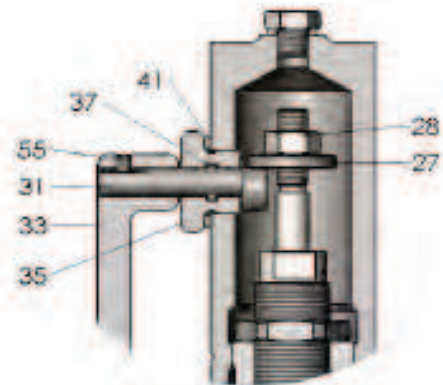
Alavanca fechada
