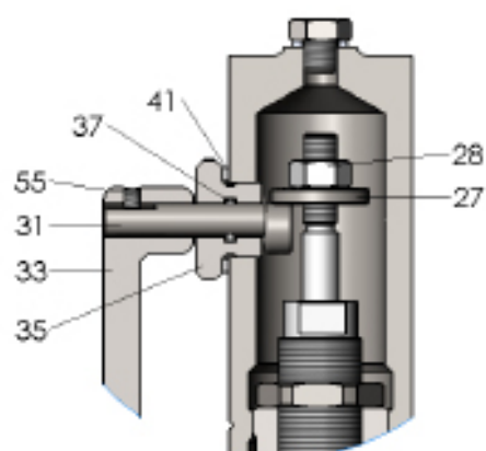
Alavanca fechada
