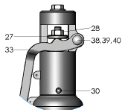
Alavanca aberta
