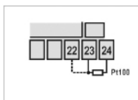
Figura 4 - conexão de Pt100 a 3 fios
