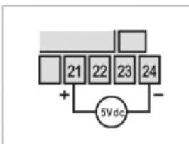
Figura 6 - conexão de tensão 0-5Vdc
