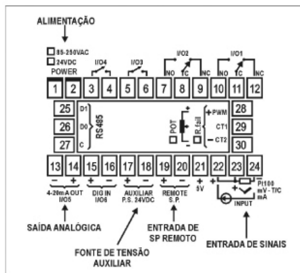
Figura 2 - Conexões do painel traseiro
